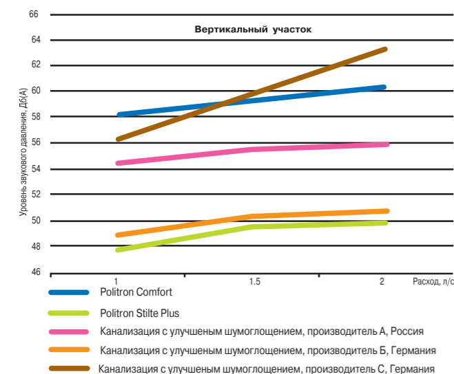
Вертикальный участок, звуковое давление, дБ(A)
