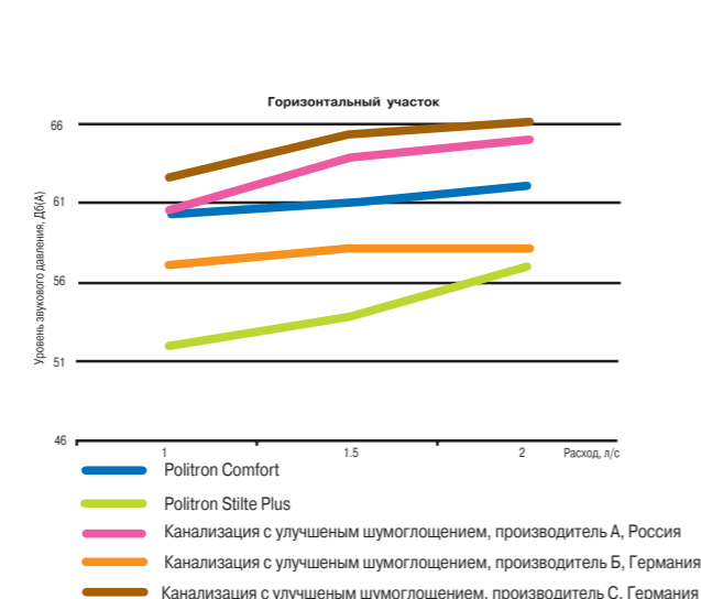
Горизонтальный участок, звуковое давление, дБ(A)
